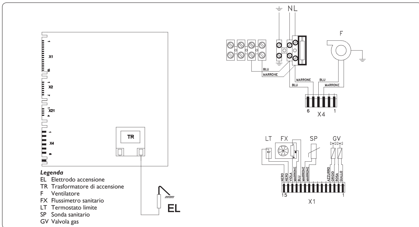
Fig. 4 - Schema elettrico
