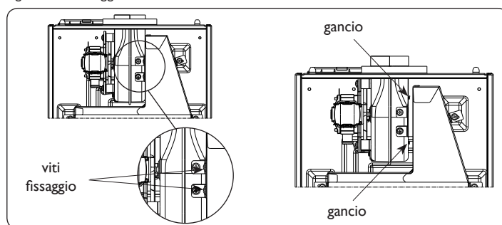
Fig. 19 - Smontaggio scambiatore
