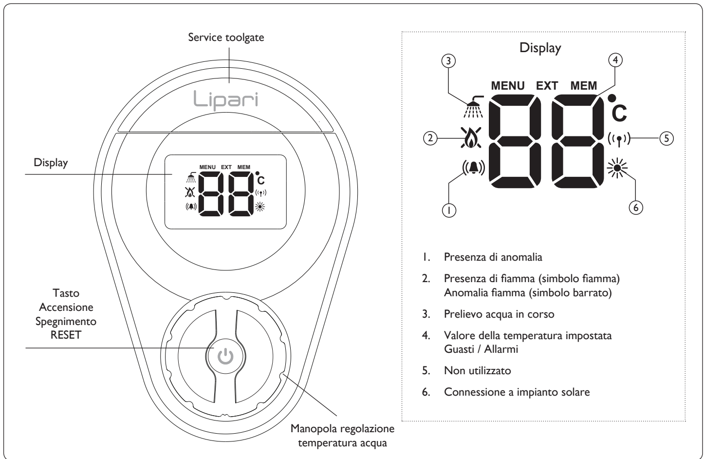
Fig. 21 - Pannello comandi e display
