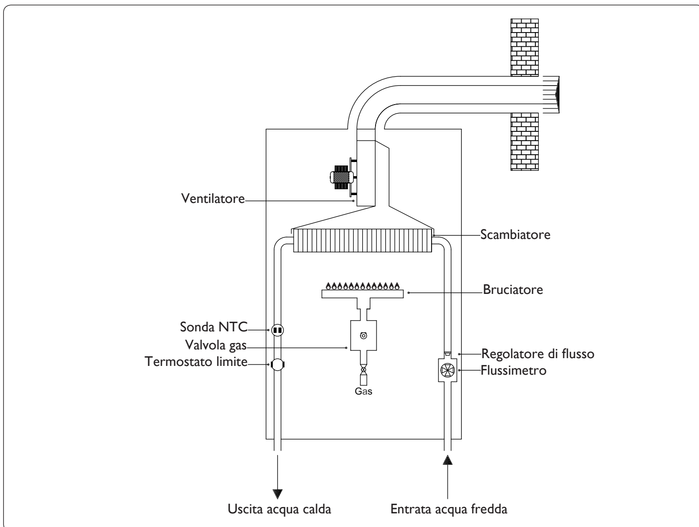
Fig. 3 - Circuito idraulico
